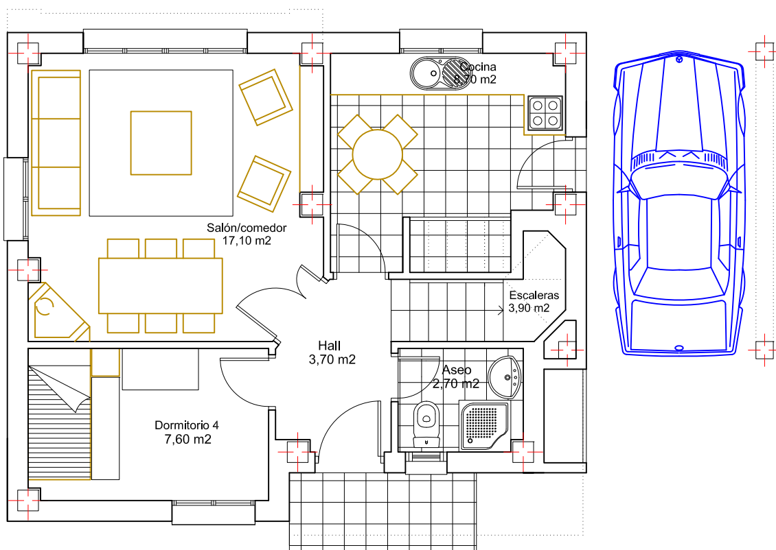
PLANTA BAJA (e:1/75)
