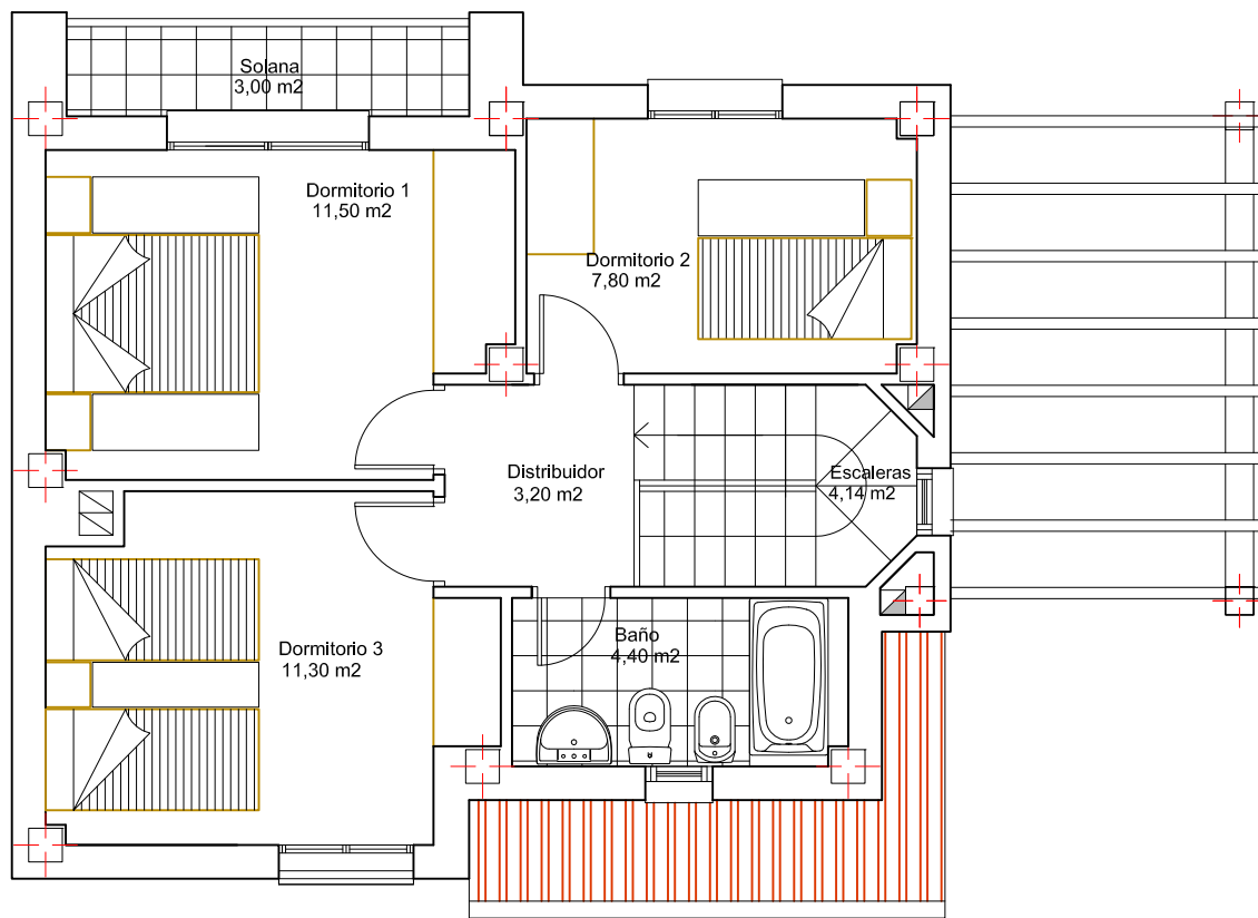
PLANTA SUPERIOR (e:1/75)
